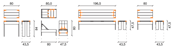
Exemples de mobilier ECH : 1/50
