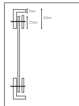
SYSTÈME DE FIXATION DES VITRINES
