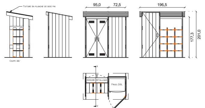
Structure principale accueillant le frigo ECH : 1/50
